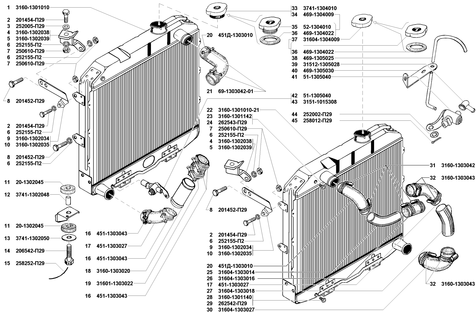
Рис. 31. Радиатор (1301) и подвеска радиатора (1302), трубопроводы и шланги (1303), пробка радиатора (1304), краник сливной (1305)
